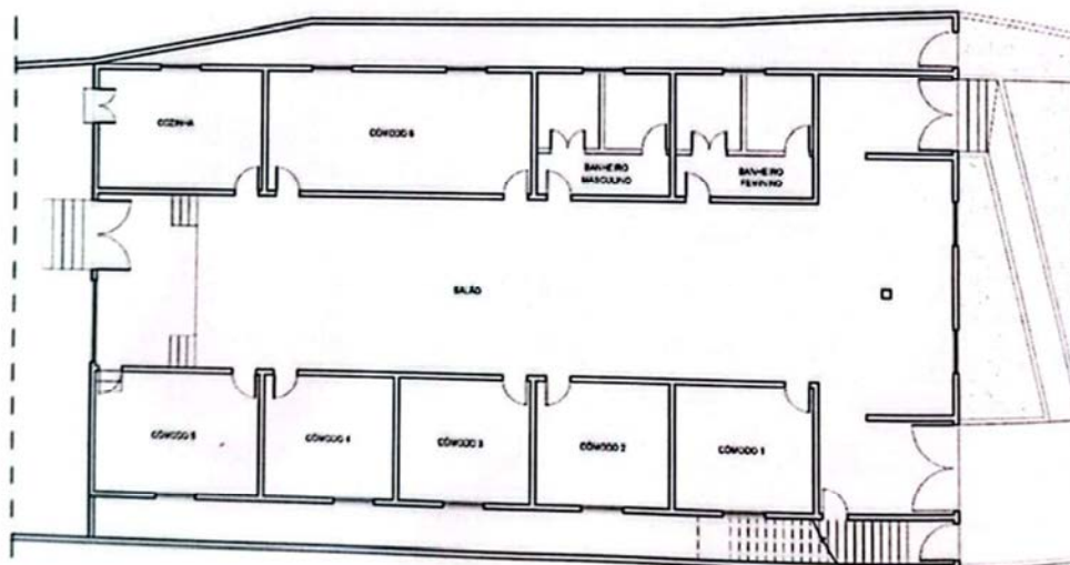
Planta da Edificação nº35 da Praça Marciano Vieira. Elaboração: Michelle Xavier. Junho/2018 Sem escala definida
